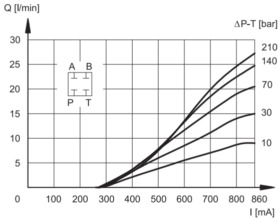
阀芯机能 C08
