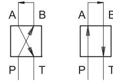
阀芯机能 A08
