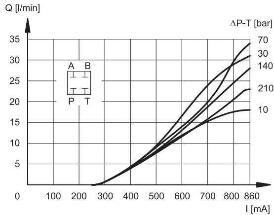
阀芯机能 C16
