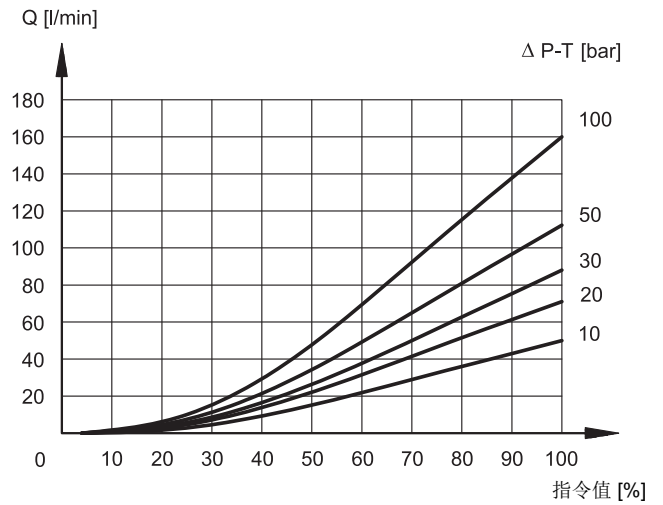
阀芯机能 Z50
