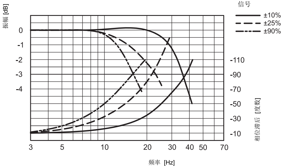
频率响应 (阀芯机能 Z - 4/3 阀)
