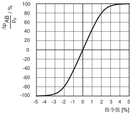
Z 阀芯机能压力增益
