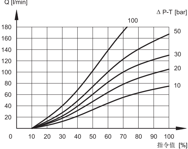
阀芯机能 A75 - C75
