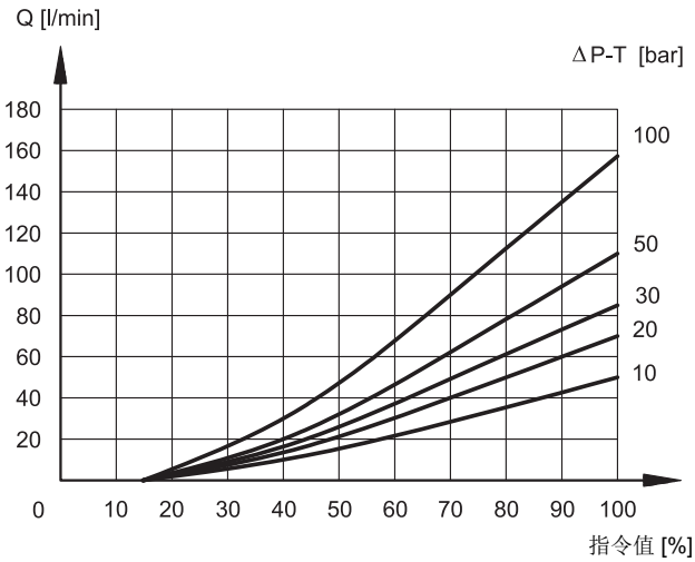
阀芯机能 A50 - C50
